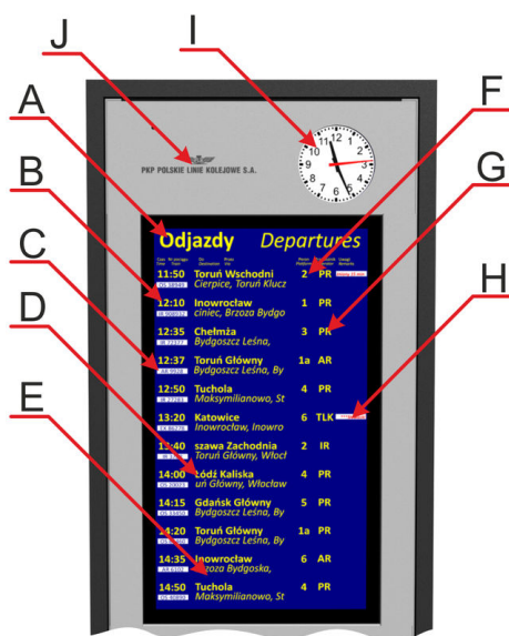
Rys. 1. Przykładowy układ informacji prezentowanych na wyświetlaczu
